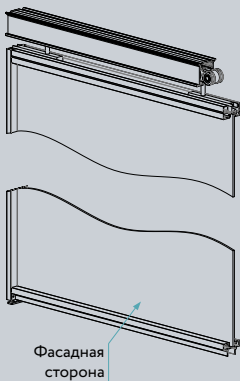
Односторонняя дверь
